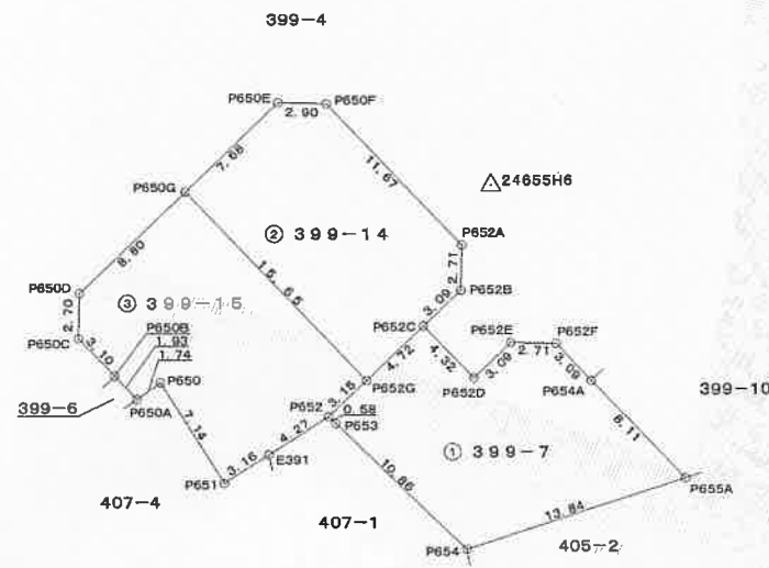
基準点詳細図 縮尺:1/30
